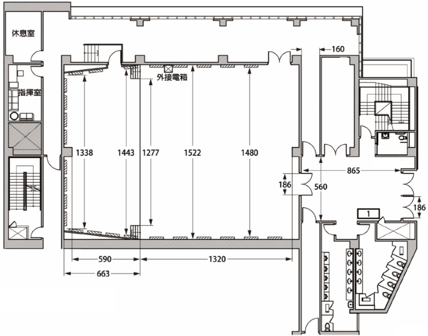
圖(一) 3201 平面圖(單位：公分)
